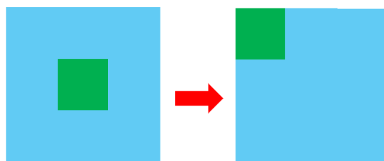
Hình 4: Hình minh họa dời “đảo cá sấu” đến góc hồ
