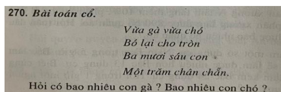
Hình 2: Ví dụ 1 bài toán giả thiết tạm
