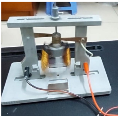
Hình 3. Mô hình động cơ Ritchie
