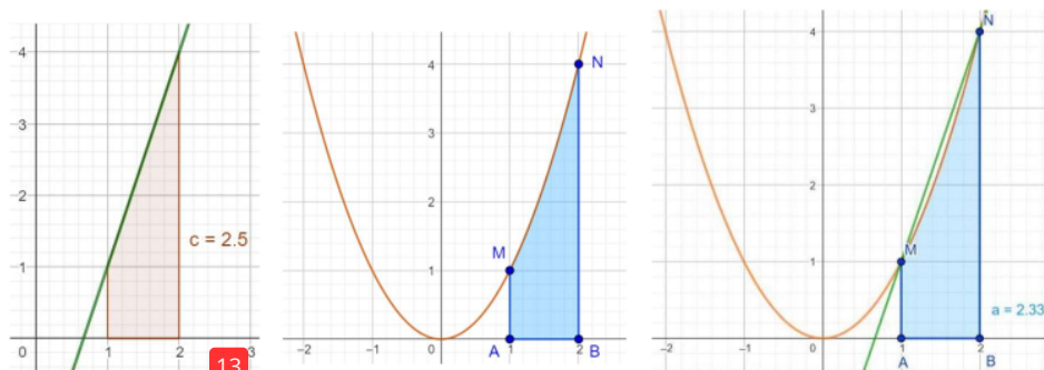
Hình 2.3. Hình phẳng giới hạn bởi đồ thị hàm số f(x) , trục Ox và x=a , x=b (câu a, câu b)
