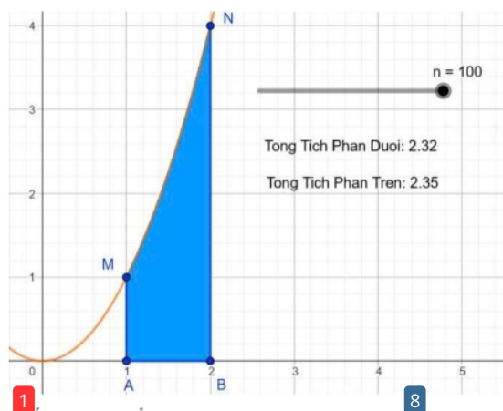
Hình 2.8. Kết quả tính tổng diện tích các hình chữ nhật trong trường hợp n = 100
