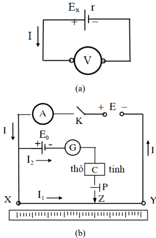
Hình 2. Sơ đồ mạch điện theo lý thuyết (a) và mạch xung đối giữa nguồn chuẩn E_0 và nguồn điện E (b).
