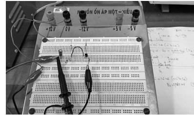
Hình 11. Mạch điện thử tải cho máy phát hàm VLQ300
