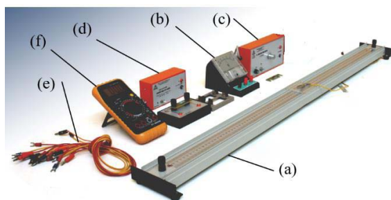
Hình 1. Bộ thí nghiệm BKE-020.
